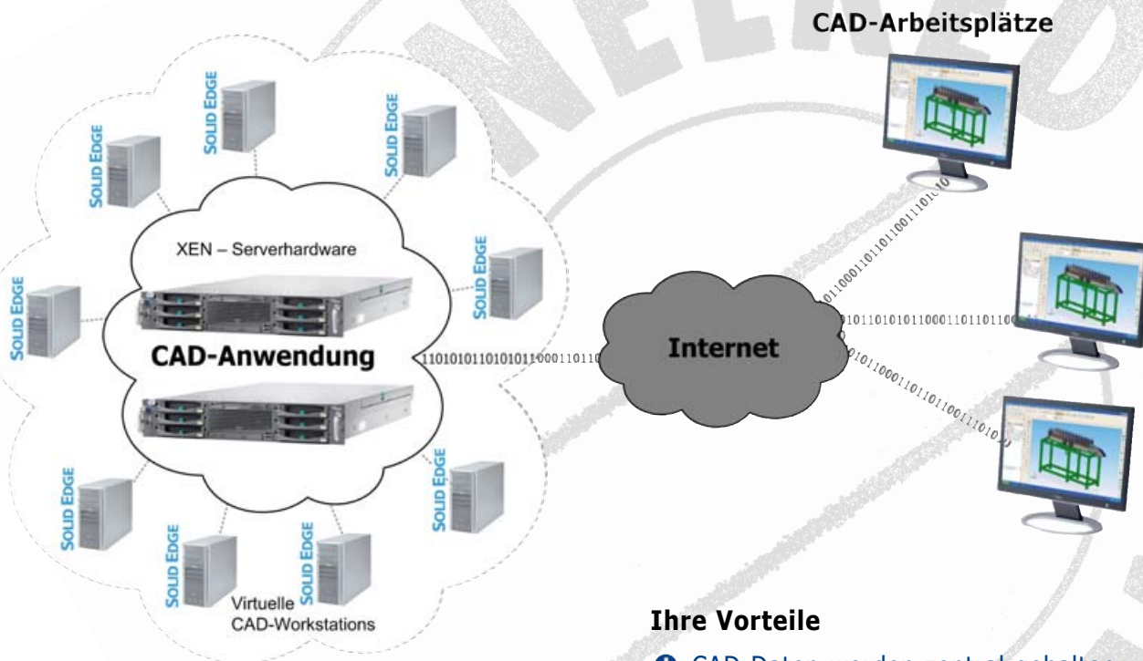
Abb. IRES-Systemaufbau
